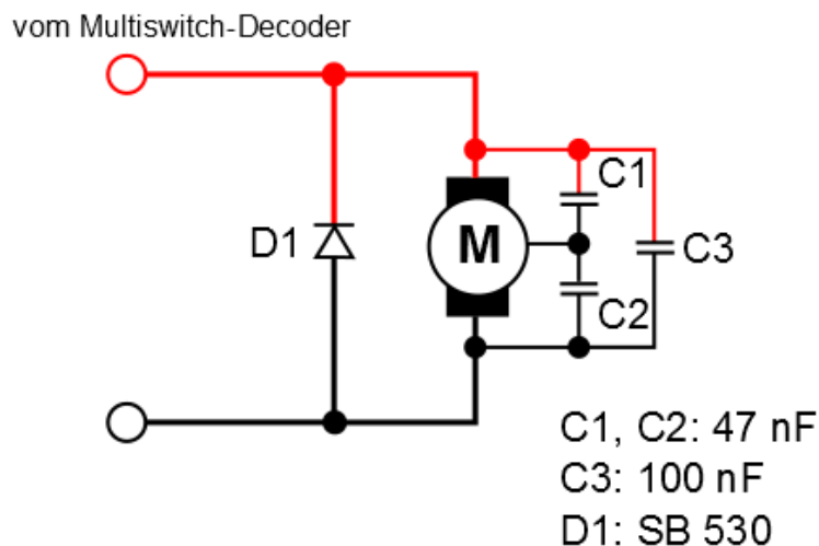
Abb. 2: Anschluss eines Motors mit Entstörkondensatoren und Freilaufdiode.
