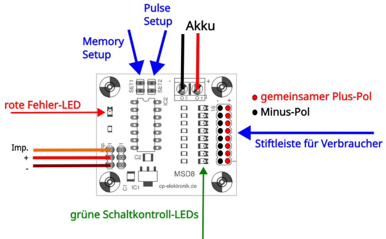
Abb.1: Anschluss des Decoders
