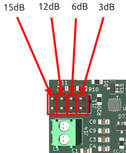
Abbildung 5: Position des Jumpers zur Einstellung der Lautstärke
