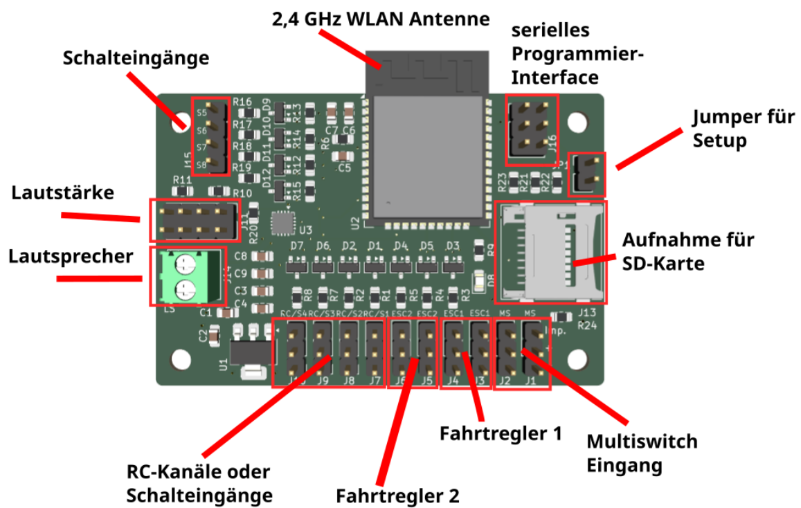
Abbildung 1: Anschlussbelegung
